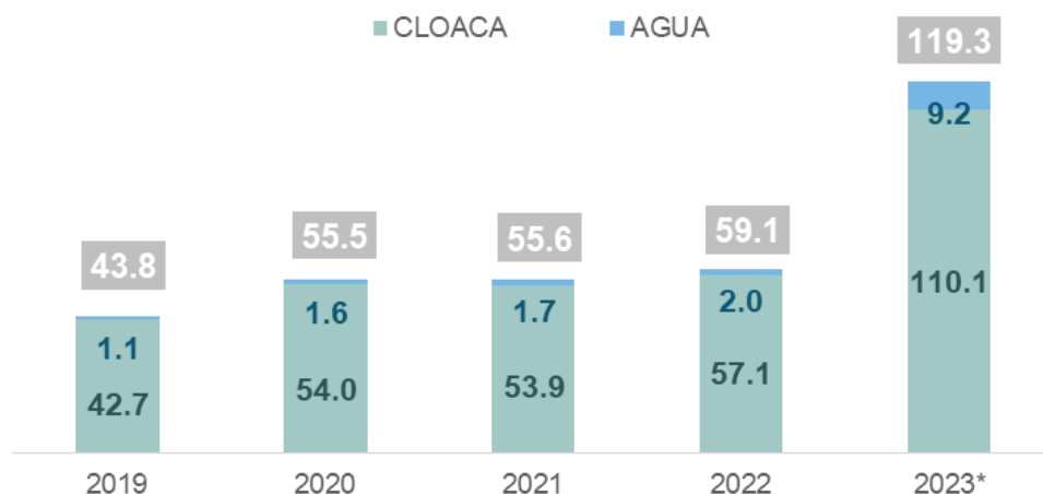
EVOLUCIÓN KM DE CAÑERÍA INSTALADA AÑO 2019 A 2023
